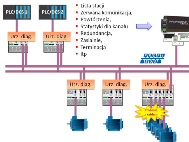
Rys. 19 – Problemy z okablowaniem lub zakłócenie komunikacji z urządzeniem mogą być wykryte przez ProfiHub i przypisane do kanału. Informacje te udostępniane są przez sieć PROFIBUS sterownikowi PLC. ProfiTrace także może odbierać te informacje.
