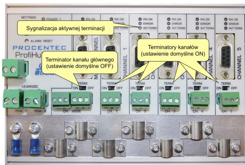
Rys. 15 – Przelączniki aktywujące terminatory.
