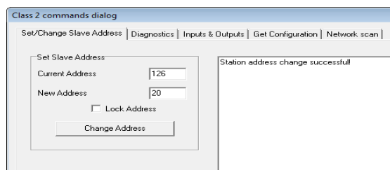
Rys. 21 – Przykład: ProfiCaptain wykorzystany do zmiany adresu z 126 na 20.
