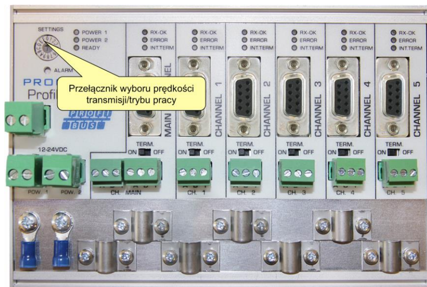
Rys. 16 – Przełącznik ustalania trybu pracy ProfiHub B5+
