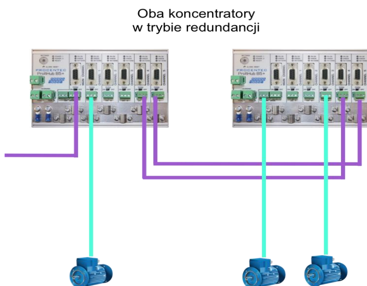
Rys. 18 - Redundantna ścieżka pomiędzy dwoma urządzeniami ProfiHub B5+.
