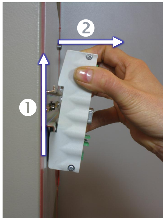
Rys. 2 Demontaż: przesunąć w górę i pociągnij
